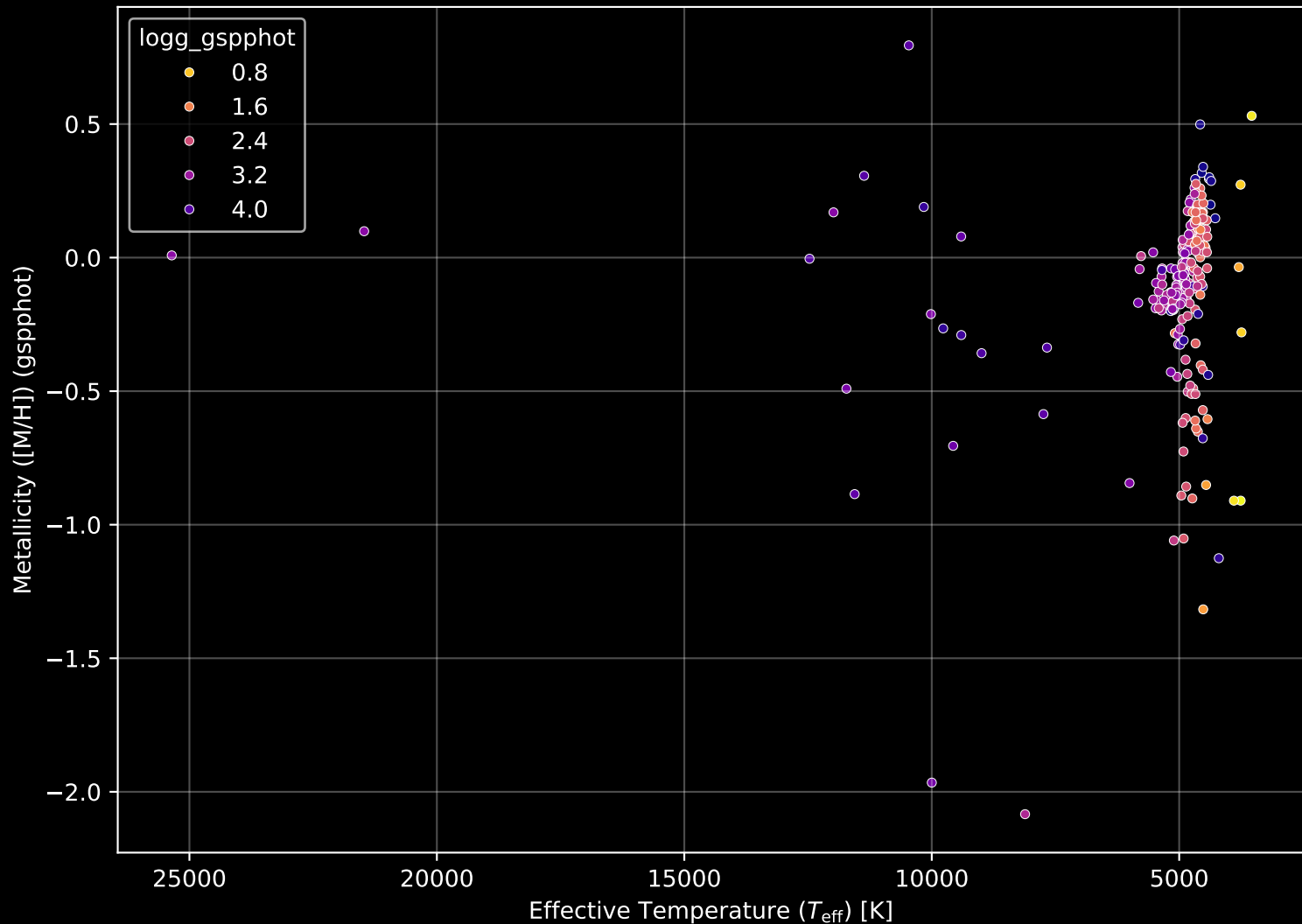
APOGEE DR17 Field: [109-08] Stellar Population Parameters (n= 238)
